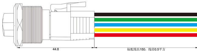
钥匙钮与连接器组合图：
